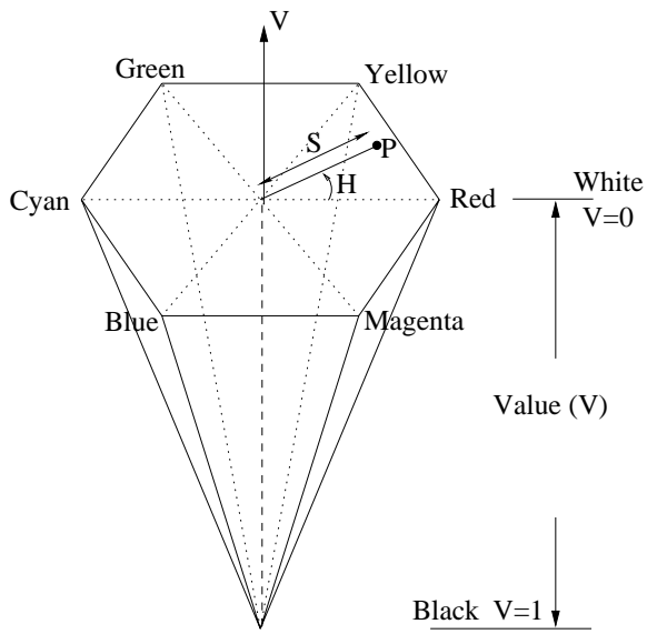
Fig. 1.12. The HSV Color Space
